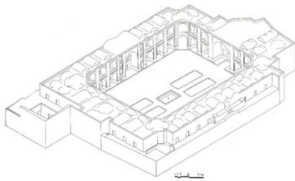
تصویر ۴: تصویر سه‌بعدی از مدرسه جده‌بزرگ (مأخذ: حاجی قاسمی، ۱۳۹۴)
