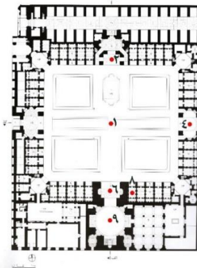
تصویر ۵: نقاط انتخاب‌شده در مدرسه چهارباغ، پلان طبقه همکف (مأخذ: حاجی قاسمی، ۱۳۹۴)
