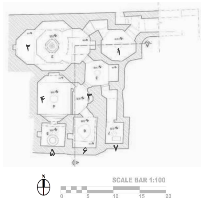
تصویر ۶: حمام تاریخی باغ فرح‌آباد. ۱- هشتی ورودی ۲- بینه و سرپینه ۳- میاندر ۴- گرم‌خانه ۵- خزینه ۶- تنظیف‌خانه ۷- سرویس بهداشتی (نسیمی، ۱۳۹۵).
