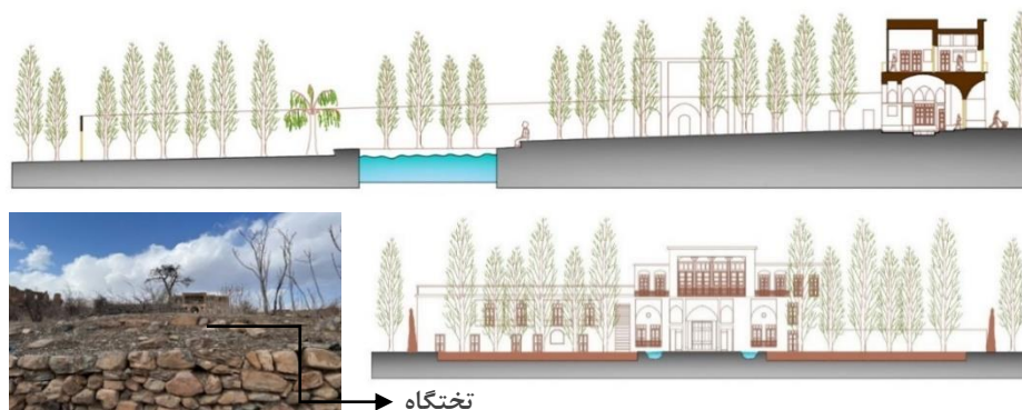
تصویر ۱۴: بالا؛ برش طولی تختگاه‌ها و استخر میان باغ بر اساس توصیفات ضربی، پایین راست؛ برش عرضی از باغ فرح‌آباد.
