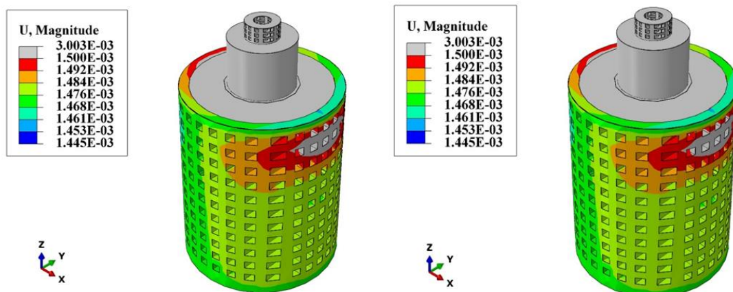
تصویر ۳۱: کانتور جابه‌جایی در مدل دارای چوب در ۴ ثانیه
