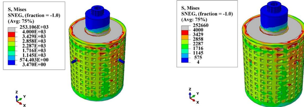
تصویر ۲۹: کانتور تغییرات تنش در مدل بدون چوب در ۴ ثانیه
