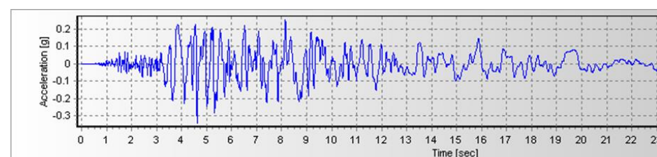
تصویر ۳: نمودار مؤلفه‌ی طولی شتاب‌نگاشت زلزله نورث ریج (مأخذ: برداشت شده توسط نگارندگان در نرم‌افزار سیسموسیگنال)
