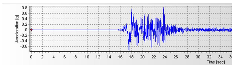
تصویر ۱: نمودار مؤلفه‌ی طولی شتاب‌نگاشت زلزله بم (مأخذ: برداشت شده توسط نگارندگان در نرم‌افزار سیسموسیگنال)
