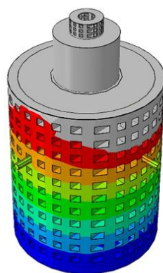
تصویر ۲۸: کانتور جابه‌جایی در تائیه ۱/۰۵۶ در مدل دارای چوب
