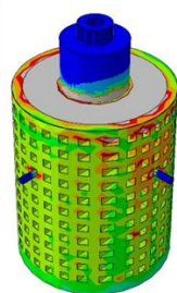
تصویر ۲۱: کانتور تغییرات تنش فون میزس در ثانیه ۴ در مدل بدون چوب تصویر ۲۲: کانتور تغییرات تنش فون میزس در ثانیه ۴ در مدل دارای چوب
