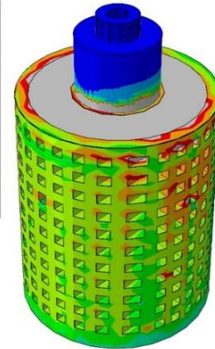
تصویر ۲۹: کانتور تغییرات تنش در مدل بدون چوب در ۴ ثانیه
