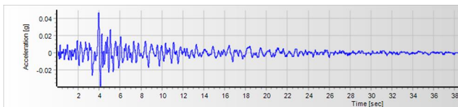
تصویر ۸: نمودار مؤلفه‌ی عرضی شتاب‌نگاشت زلزله دریچه کیوته (مأخذ: برداشت‌شده توسط نگارندگان در نرم‌افزار سیسموسیگنال)
