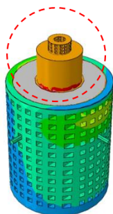
تصویر ۲۱: کانتور تغییرات تنش فون میزس در ثانیه ۴ در مدل بدون چوب تصویر ۲۲: کانتور تغییرات تنش فون میزس در ثانیه ۴ در مدل دارای چوب
