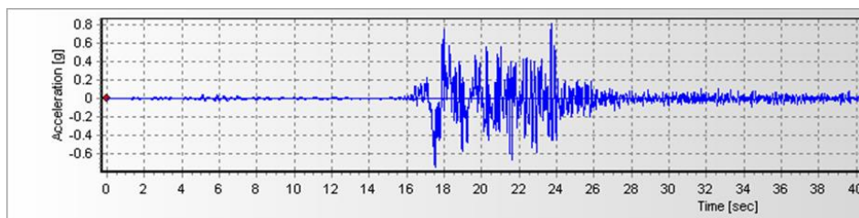
تصویر ۴: نمودار مؤلفه‌ی طولی شتاب‌نگاشت زلزله دریچه کیوته (مأخذ: برداشت‌شده توسط نگارندگان در نرم‌افزار سیسموسیگنال)
