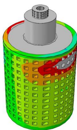
تصویر ۳۱: کانتور جابه‌جایی در مدل دارای چوب در ۴ ثانیه
