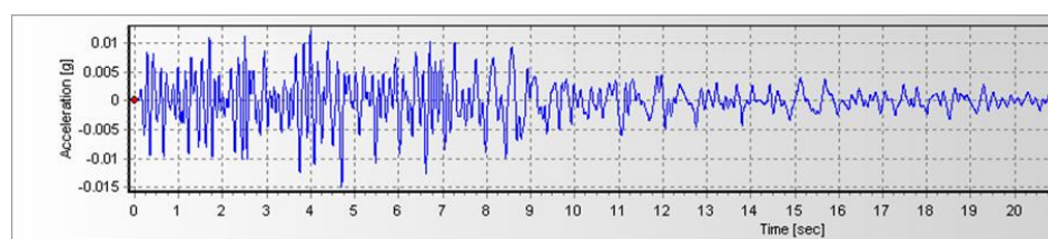
تصویر ۲: نمودار مؤلفه‌ی طولی شتاب‌نگاشت زلزله ایمپریال ولی (مأخذ: برداشت شده توسط نگارندگان در نرم‌افزار سیسموسیگنال)
