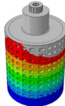
تصویر ۲۷: کانتور جابه‌جایی در تائیه ۱/۰۵۶ در مدل بدون چوب
