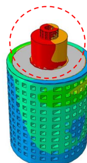
تصویر ۲۳: کانتور جابه‌جایی در ثانیه ۳/۸۵۶ تصویر ۲۴: کانتور جابه‌جایی در ثانیه ۳/۸۵۶
