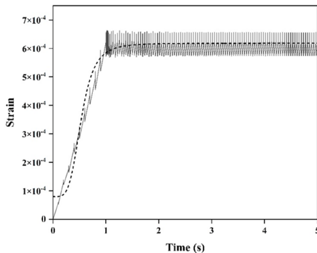
تصویر ۴۳: نمودار تغییرات کرنش حقیقی- زمان در مدل دارای چوب در زلزله دریاچه کیوته
