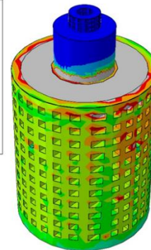
تصویر ۲۵: کانتور تغییرات تنش فون میزس در تائیه ۴ در مدل بدون چوب
