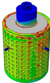
تصویر ۲۶: کانتور تغییرات تنش فون میزس در تائیه ۴ در مدل دارای چوب
