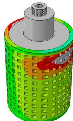
تصویر ۳۰: کانتور جابه‌جایی در مدل بدون چوب در ۴ ثانیه
