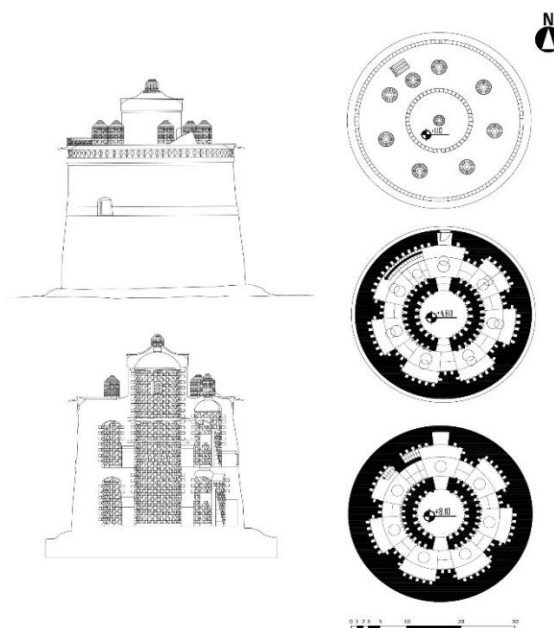
تصویر ۱۴: پلان برج استوانه‌ای (گونه ۴).
