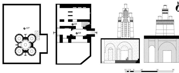
تصویر ۱۷: پلان برج چهار استوانه (گونه ۶).
