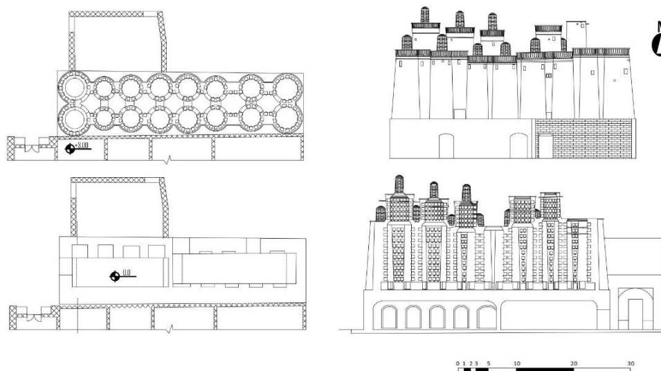
تصویر ۲۱: پلان برج مجموعه چند استوانه‌ای (گروه ۷).
