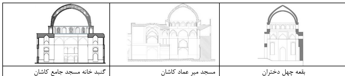
شکل ۱۴. ستون از راست به چپ: بالا؛ طرح شماتیک ساخت گنبدخانه، پایین؛ محراب گنبدخانه، بالا؛ نمایی از گنبدخانه مسجد جامع، پایین؛ بقعه چهل دختران، بالا؛ ایوان مسجد جامع، پایین؛ تزئینات ایوان مسجد بابولی و ردیف آخر؛ از چپ به راست، مقطع گنبدخانه مسجد جامع کاشان، مسجد میرعماد کاشان، بقعه چهل دختران کاشان
