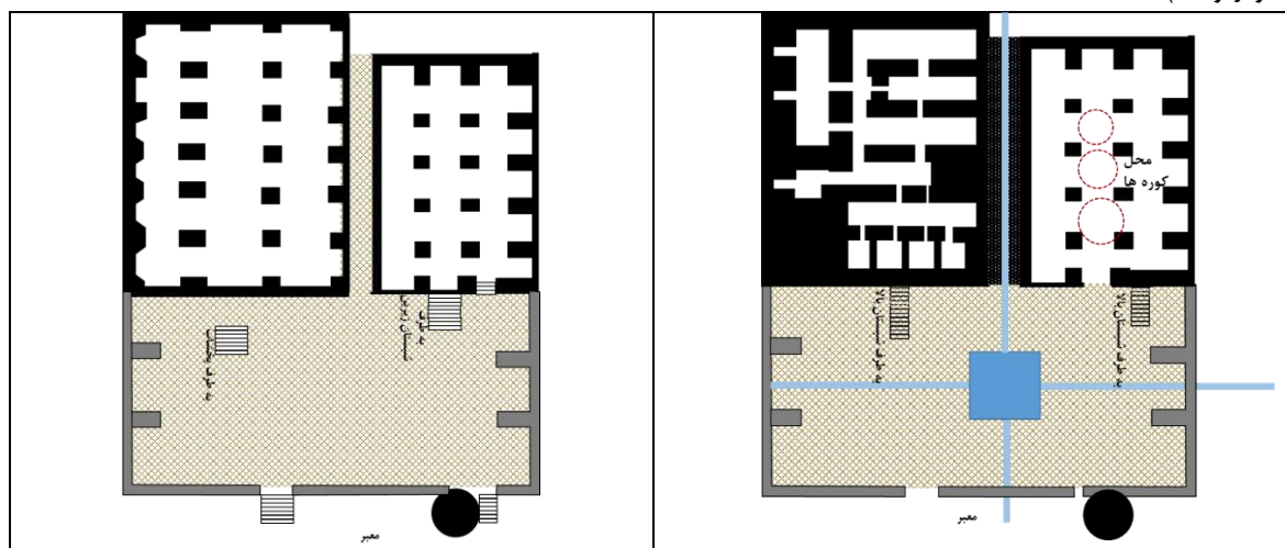
شکل ۱۲. سمت راست: طرح شماتیک فرضیه اول از طبقه ورود به مسجد (با نمایش تقریبی محل کوره‌ها و پخش‌اب)، سمت چپ: طرح شماتیک طبقه دوم از طبقه ورود به مسجد
