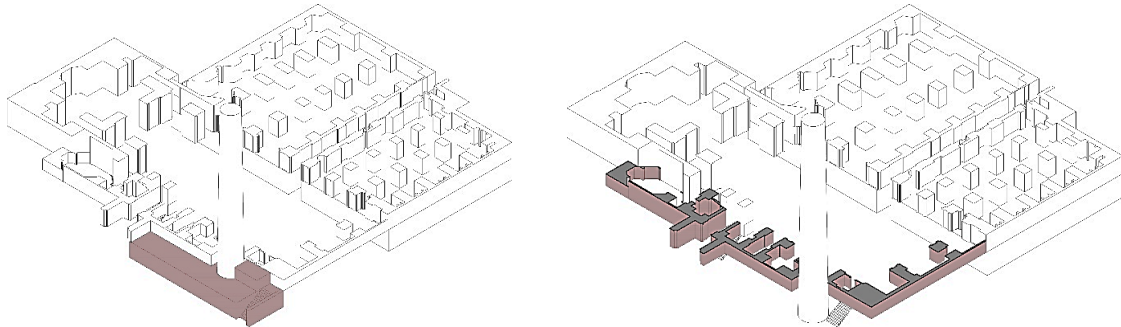
شکل ۱۶. از راست به چپ: مرحله پنجم؛ طرح شماتیک ساخت دیواره‌های پیرامون مسجد، مرحله ششم؛ ساخت مغازه در جداره بیرونی.
