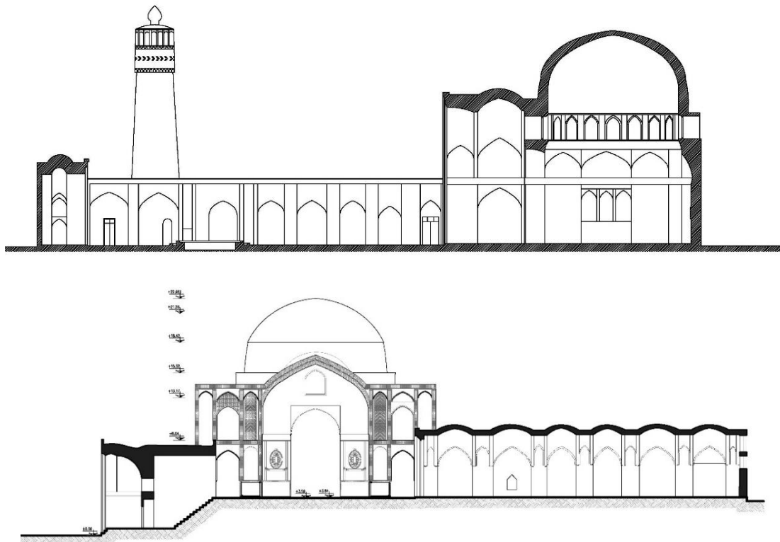
شکل ۵. بالا: برش افقی از حیاط (اداره میراث فرهنگی کاشان)، پایین: برش عمودی از حیاط (اصلاحات نگارندگان بر روی نقشه میراث فرهنگی کاشان)
