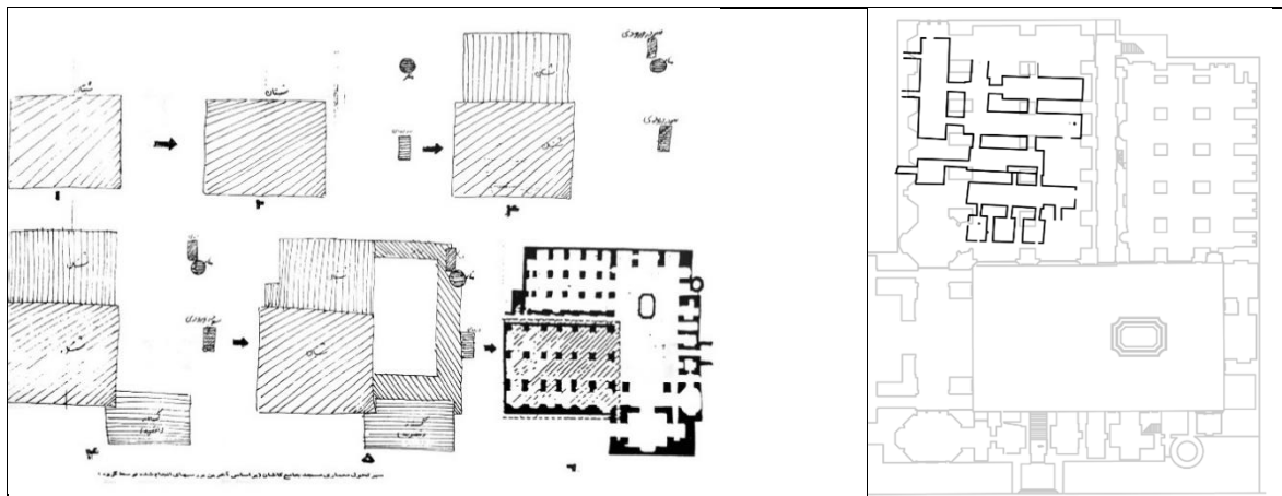
شکل ۸. سمت راست: پلان برداشت شده شبستان زیرین (ساروخانی، ۱۳۹۱). سمت چپ: توسعه و گسترش مسجد، آیت الله زاده شیرازی و همکاران (ارجمندفر، ۸۷: ۲۵۹)
