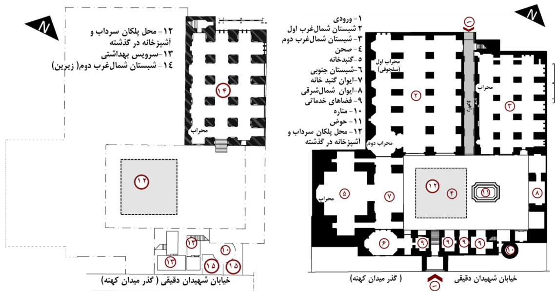
شکل ۴. سمت راست: پلان طبقه همکف، سمت چپ: پلان طبقه زیرزمین (اصلاحات نگارندگان بر روی نقشه های موجود در اداره میراث فرهنگی شهرستان کاشان)
