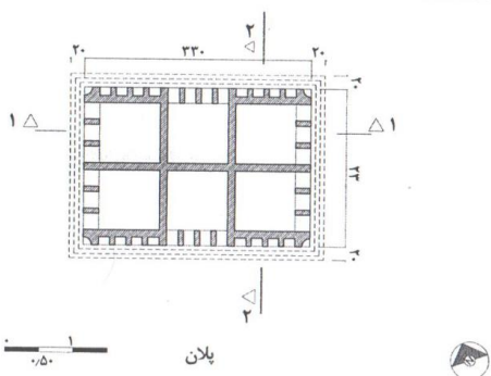
تصویر ۹- سمت چپ: جهت گیری بادگیر خانه مرتاض نسبت به محور شمال جنوب (ماخذ: محمودی، ۱۳۸۸)، راست: تصاویری از جبهه های طولی و عرضی بادگیر مورد مطالعه و تعداد منافذ باز در دهانه ورودی باد (ماخذ: نگارندگان)
