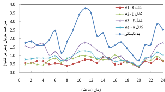
تصویر (b) ۷- میانگین تغییرات جریان هوای داخل بادگیرمراض در گرم‌ترین روز سال (ماخذ: نگارندگان)
